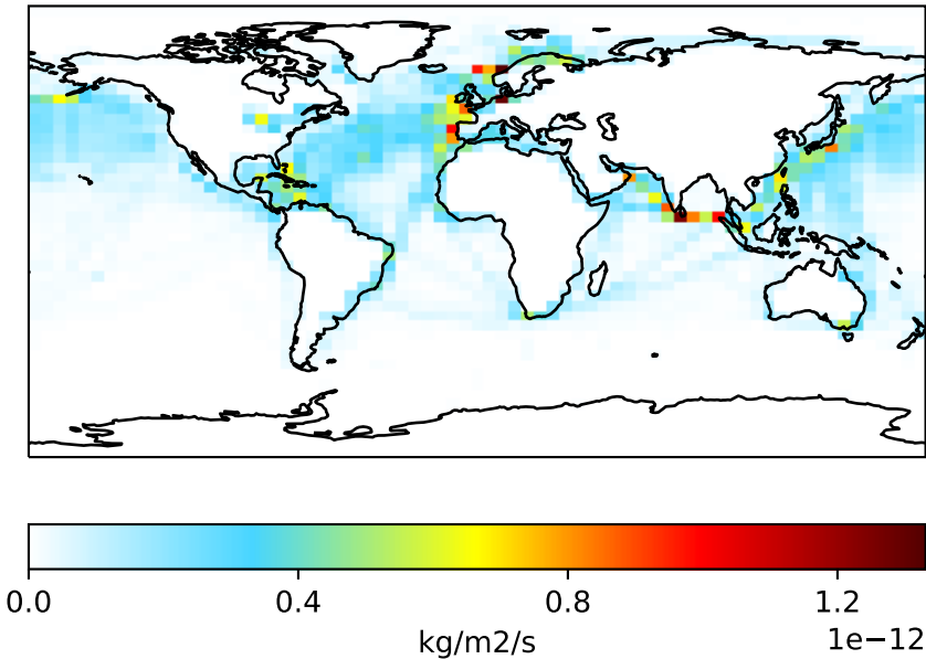
GCC_13.0.0-offlineEmis (Dev) 4.0x5.0
