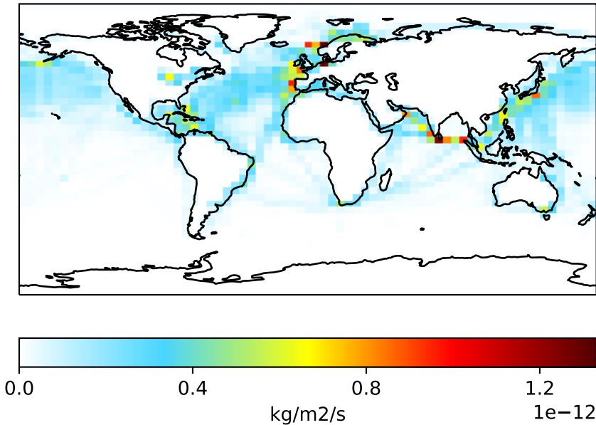
GCC_13.0.0-beta.0 (Ref) 4.0x5.0
