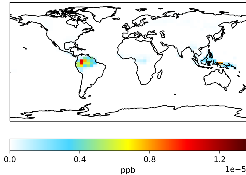
GCC_13.0.0-offlineEmis (Ref) 4.0x5.0
