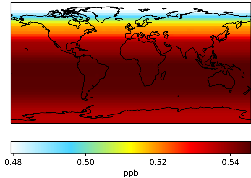
GCC_13.2.0-beta.0-LuoWetdep (Dev) 4.0x5.0
