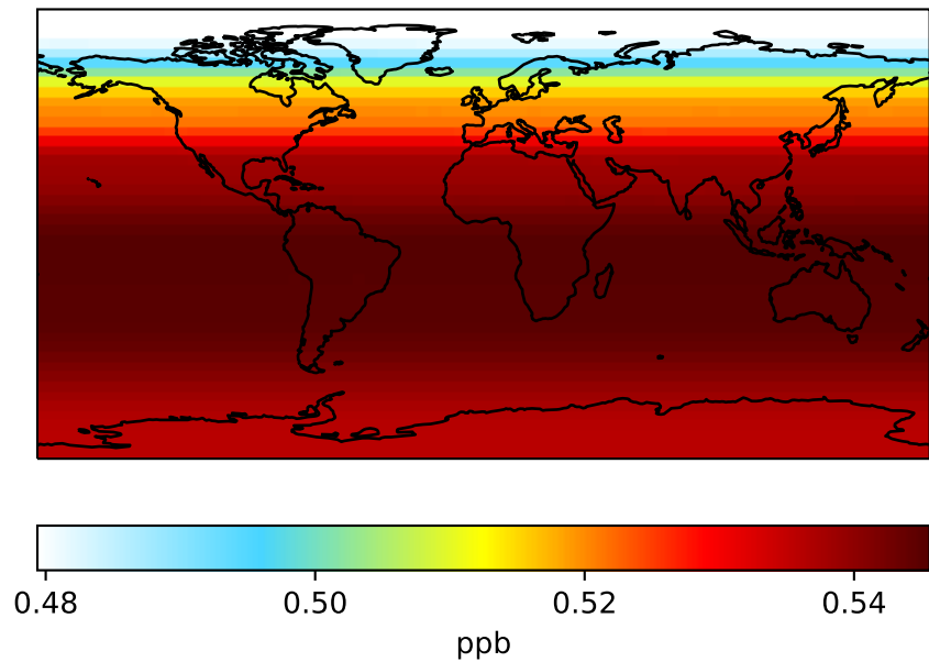
GCC_13.2.0-beta.0 (Ref) 4.0x5.0
