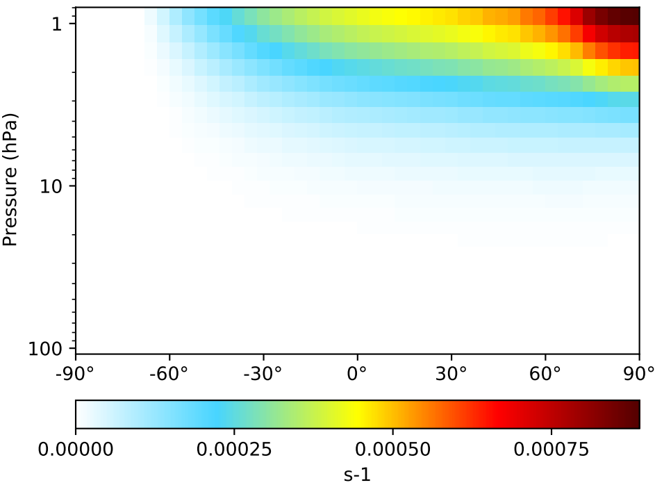
GCC_13.2.0-beta.0 (Ref) 4.0x5.0
