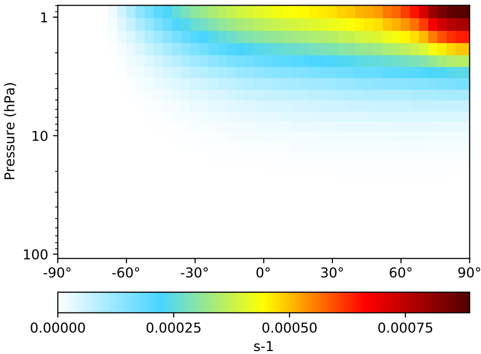
GCC_13.2.0-beta.0-LuoWetdep (Dev) 4.0x5.0
