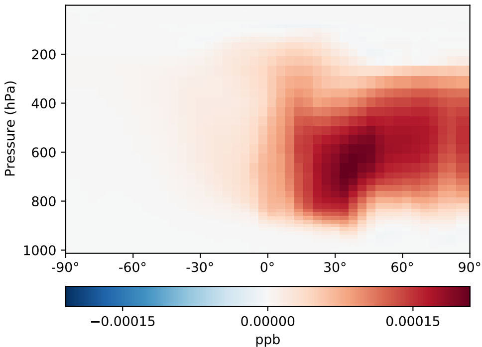
GCC_13.2.0-beta.0-LuoWetdep - GCC_13.2.0-beta.0 (Ref) 4.0x5.0 GCHP_13.2.0-beta.0-LuoWetdep - GCHP_13.2.0-beta.0 (Dev) 1x1.25 regrided from c48
