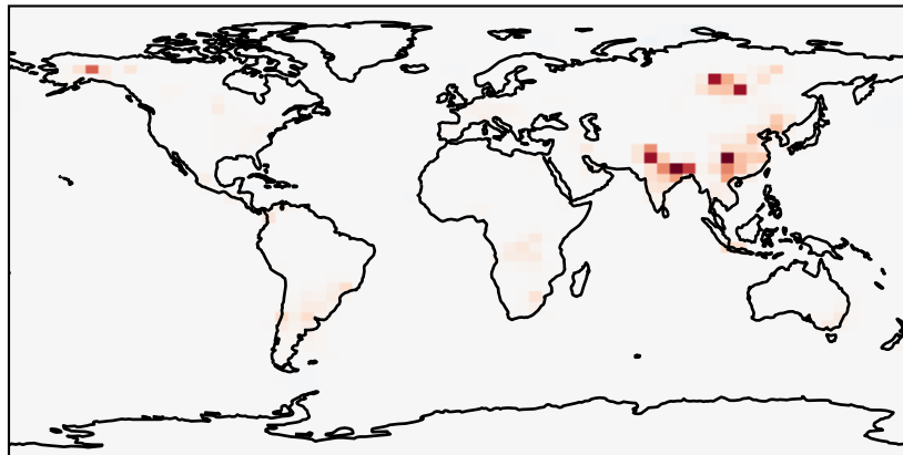
GCC_13.4.0-rc.0 - GCC_13.3.0-rc.1 (Ref) 4.0x5.0
