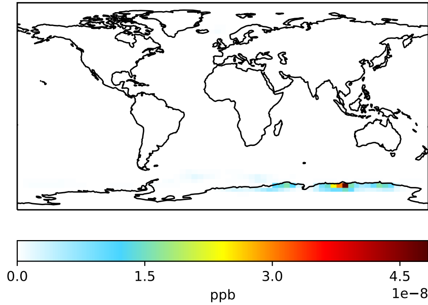
GCC_13.0.0-beta.1 (Ref) 4.0x5.0
