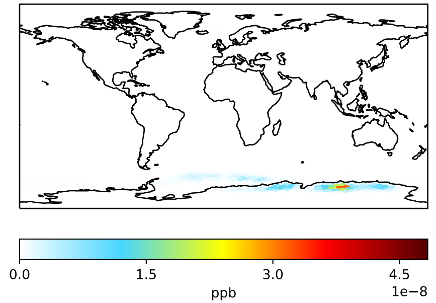
GCHP_13.0.0-beta.1 (Dev) c48
