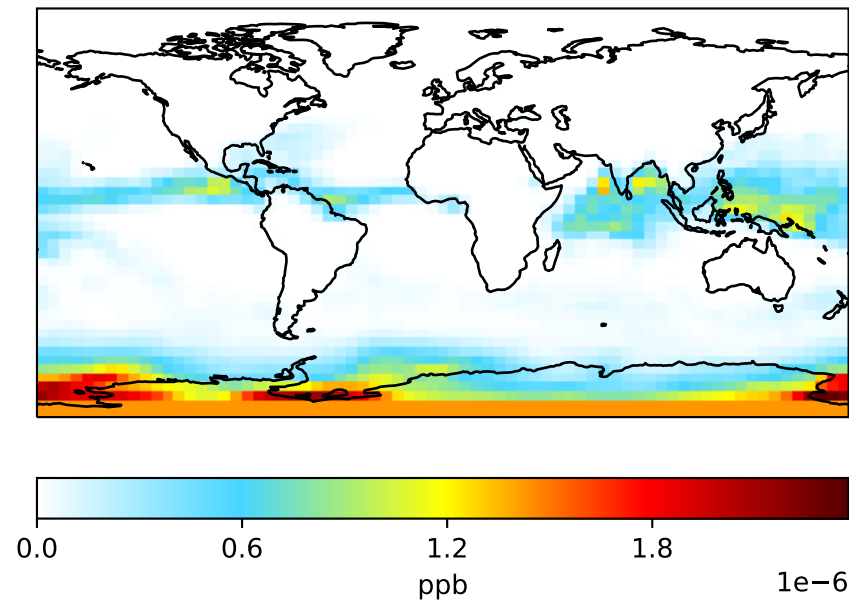
GCC_13.2.0-LuoWetdep (Dev) 4.0x5.0
