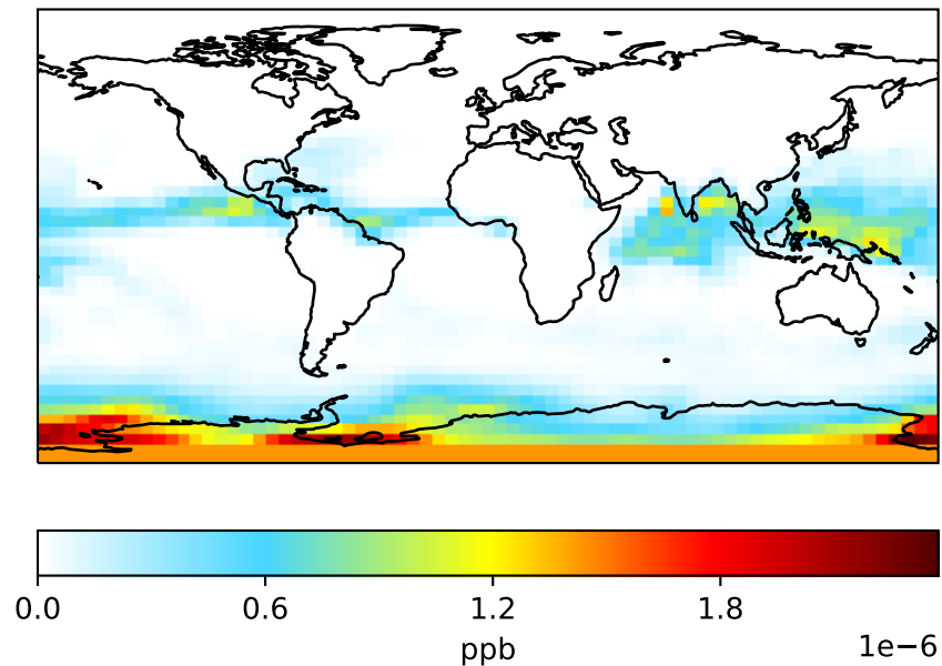
GCC_13.2.0 (Ref) 4.0x5.0
