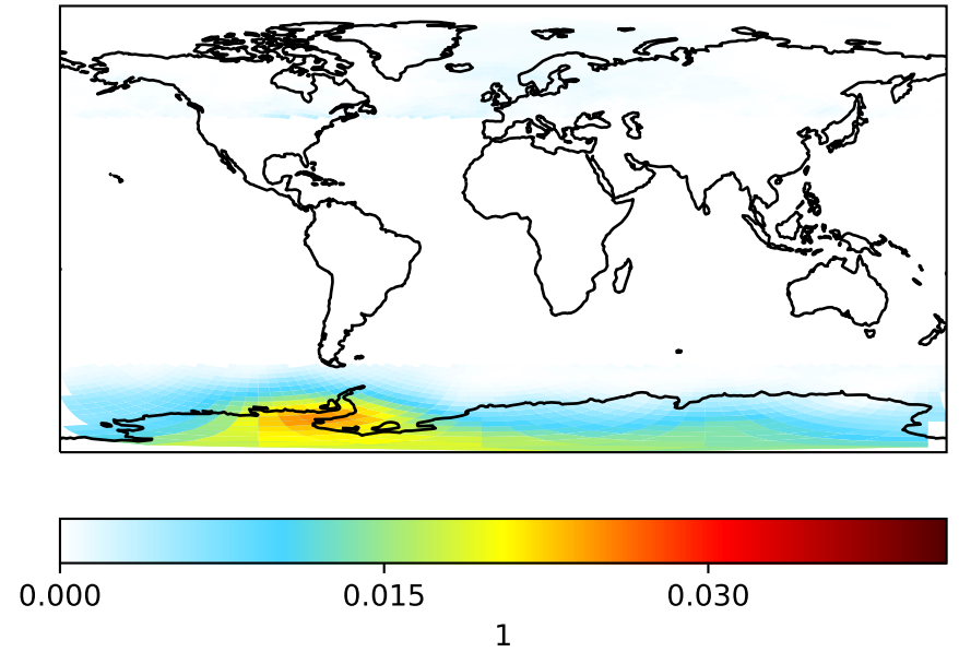
GCHP_13.2.0-LuoWetdep (Dev) c48
