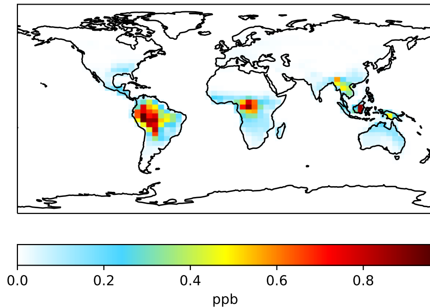
GCC_13.2.0-LuoWetdep (Ref) 4.0x5.0
