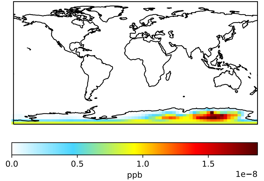
GC_12.4.0 (Dev) 4x5
