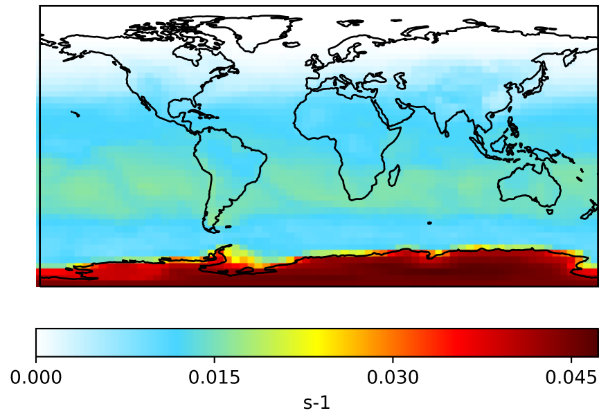
GC_12.4.0 (Ref) 4x5
