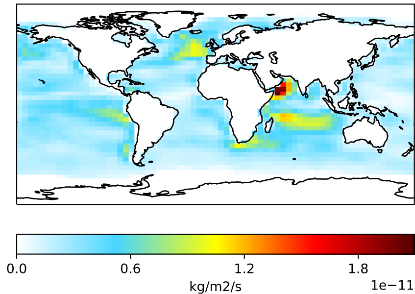
GCC_14.2.0_MERRA2 (Ref) 4.0x5.0
