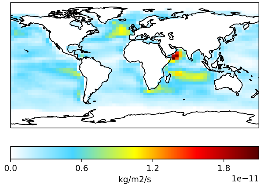
GCC_14.2.0_GEOS-IT (Dev) 4.0x5.0
