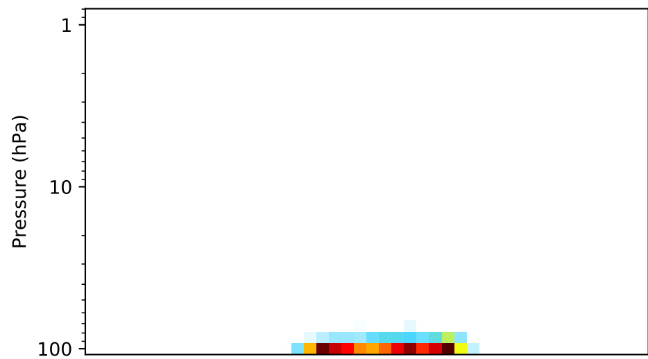
Run1-LuoWetDep (Dev) 4x5
