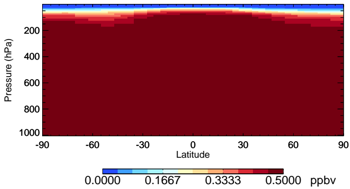
v11-02f-Run1 OCS - Species Zonal Mean for Jul
